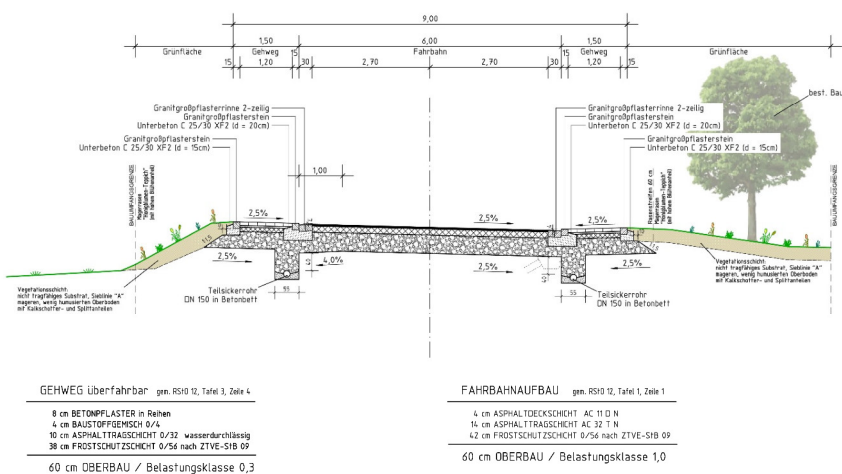
Strassenquerschnitt 1 Coburger Straße
