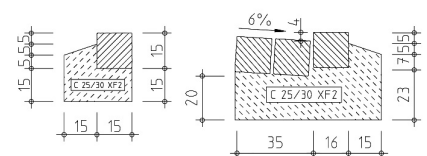
DETAIL BETONAUFLAGER
