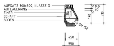
DETAIL STRASSENABLAUF
